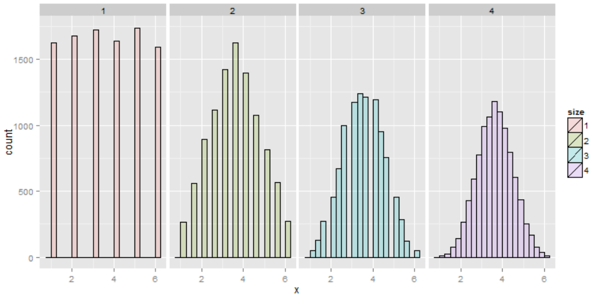
Simulation of die rolls
